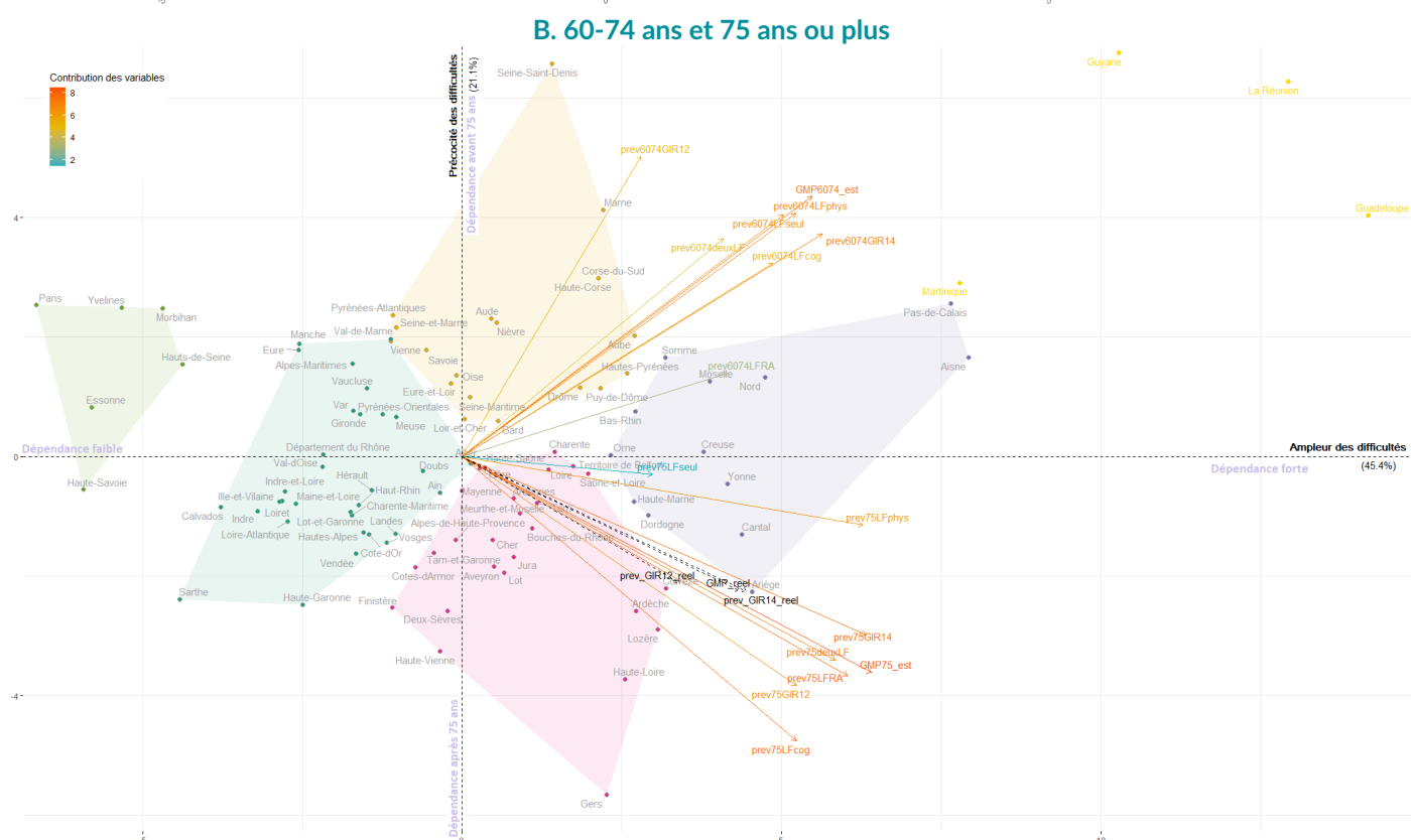
Graphique 4 – Analyse en composantes principales de la perte d'autonomie des personnes âgées de 60 ans ou plus par département en France.
